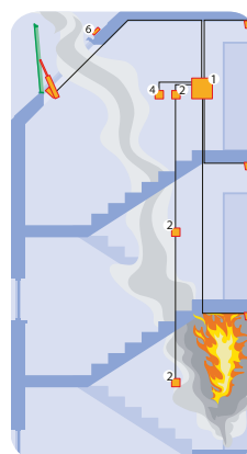
A füstelvezető rendszer működési elve
